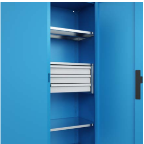
Türenverstärkung für hohe Türstabilität mit verdeckten Schließstangen
